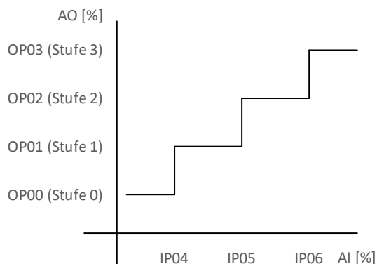
Abbildung 1: Funktion Stufen-Betrieb
