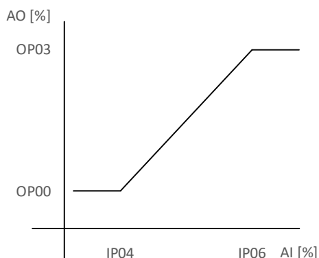
Abbildung 3: Funktion Stufenlos-Betrieb
