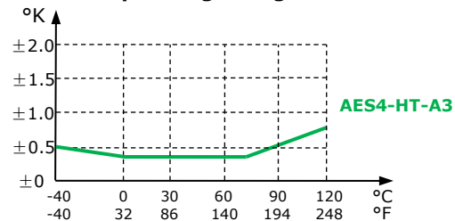
Abbildung 2: Maximale Temperatur-Toleranz
