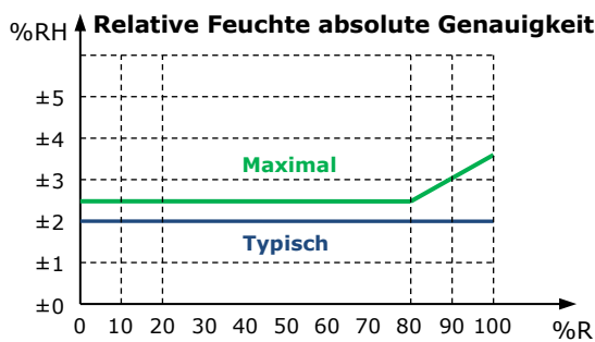
Grafik 2: Max RH-Toleranz bei 25°C (77°F) pro Sensortyp
