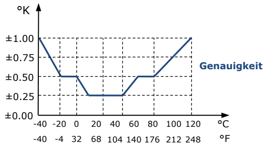
Grafik 1: Max. T-Toleranz bei Sensortyp
