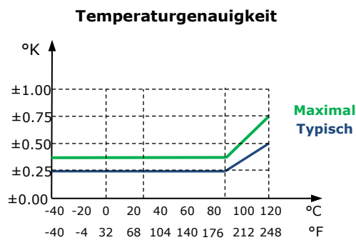
Grafik 3: Max T-Toleranz bei Sensortyp
